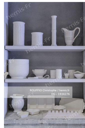
HEMIS_1934276
