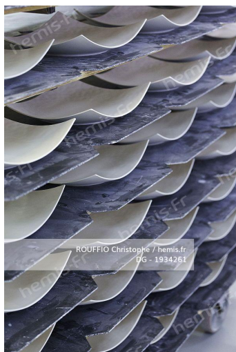
HEMIS_1934261
